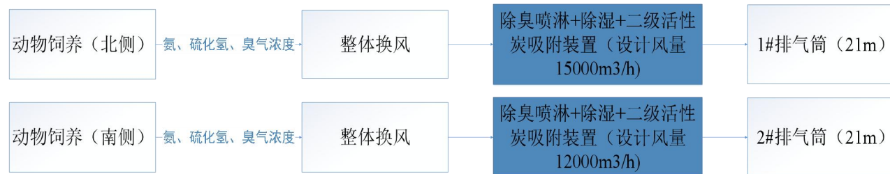
图 4-1 本项目废气处理流程图
