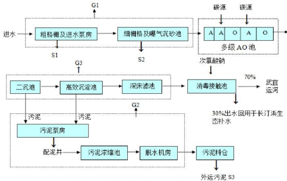
图 4-3 滨湖污水处理厂工艺流程图
